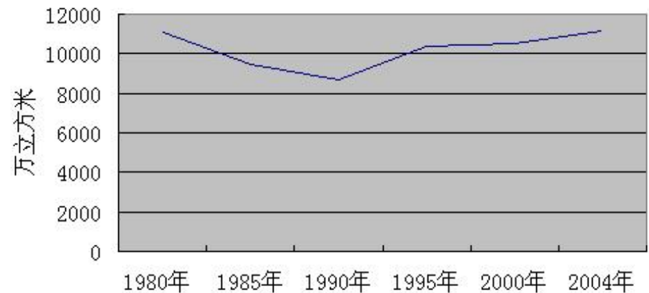
吉林省林业局天然林立木蓄积图
